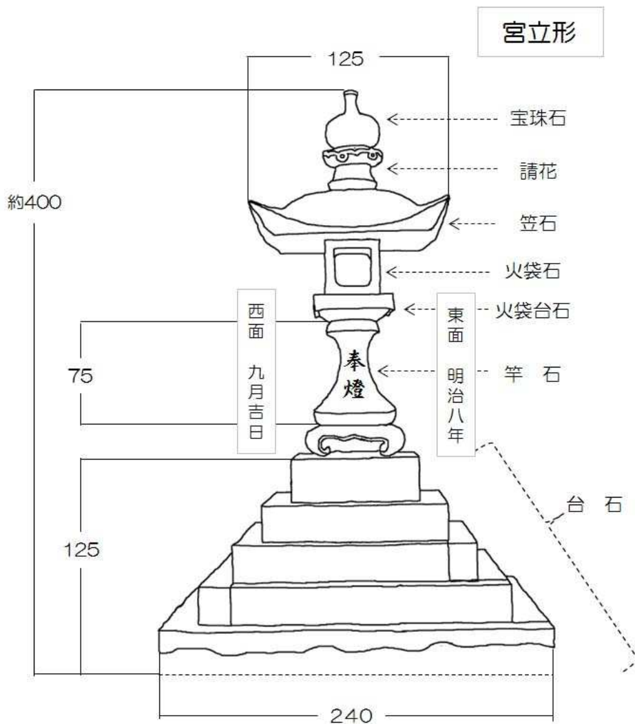
常夜燈寸法図（単位：cm）
