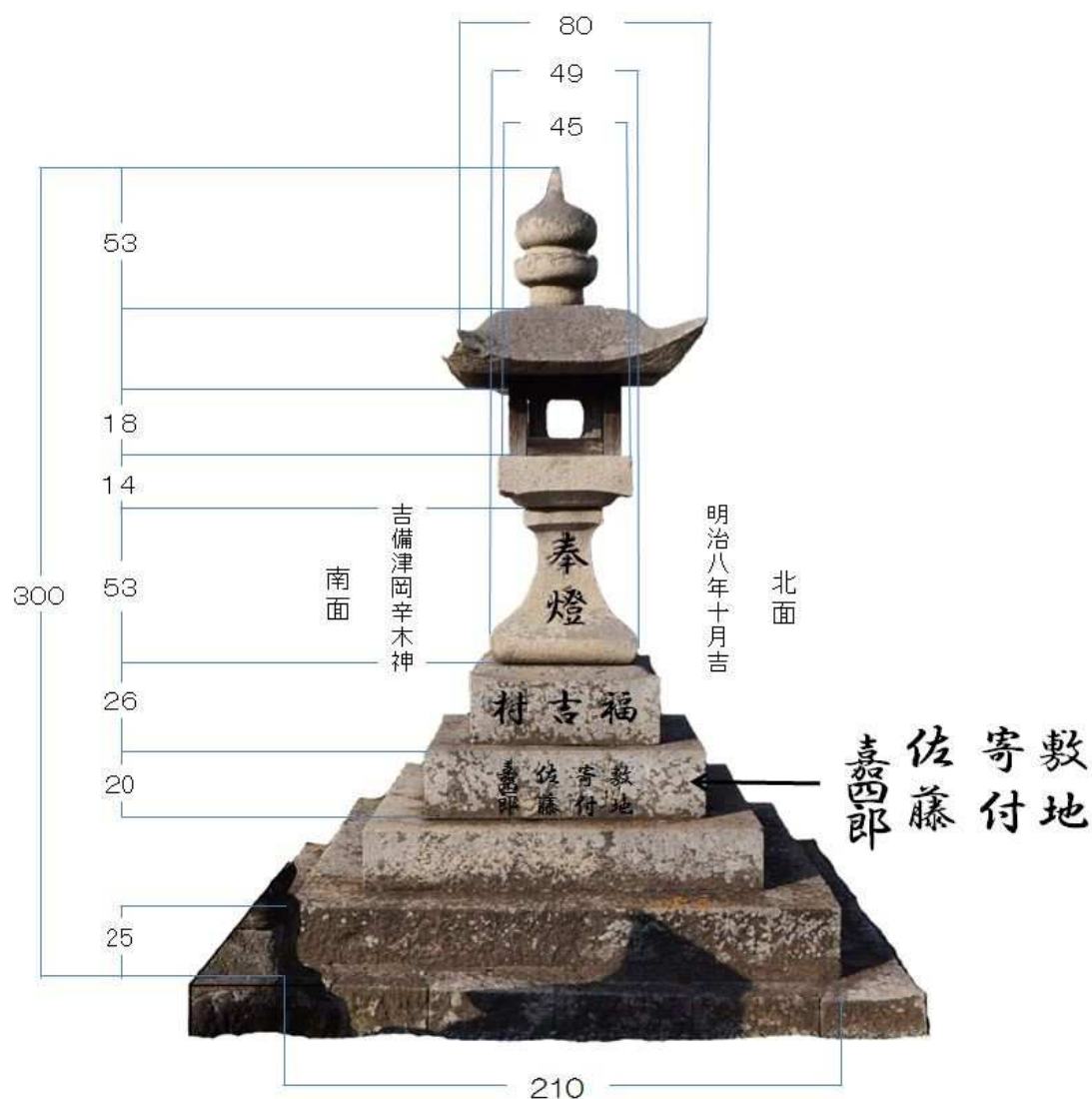
常夜燈寸法図（単位：cm）
