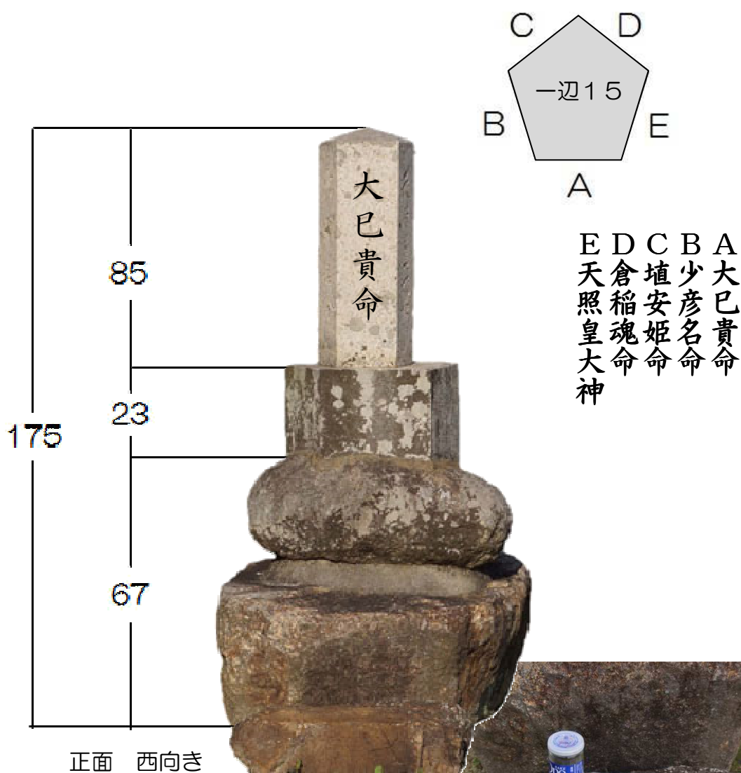
中村地神様寸法図（単位：cm）
