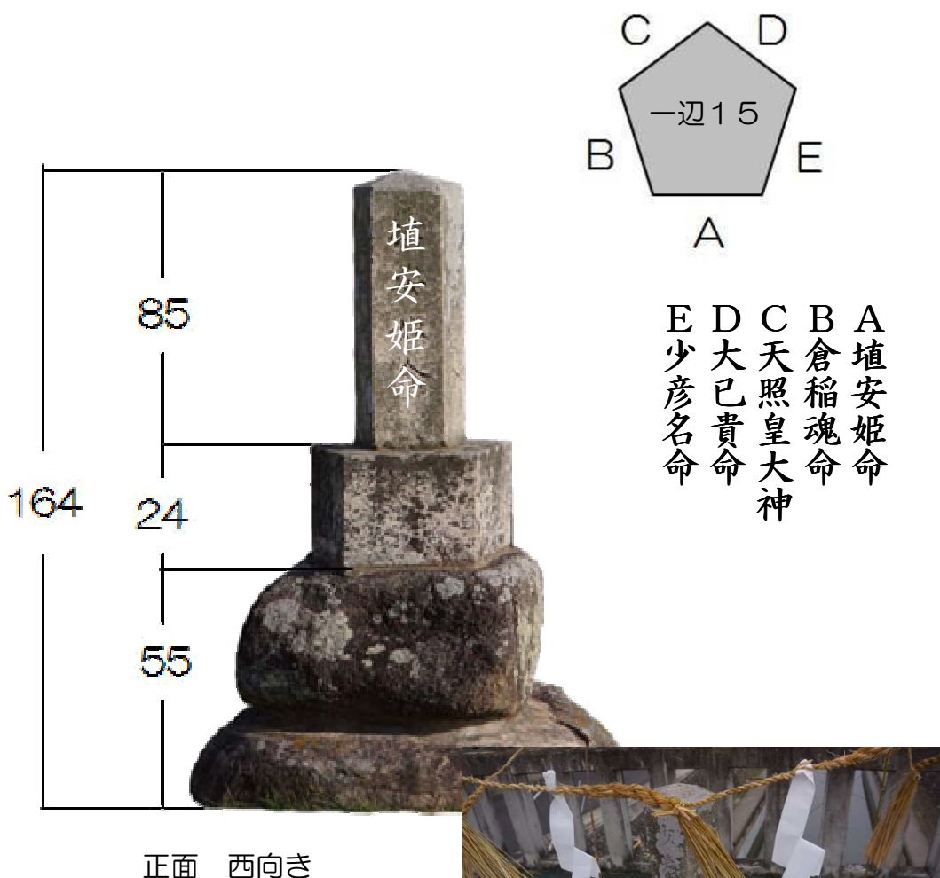
本村地神様寸法図（単位：cm）
