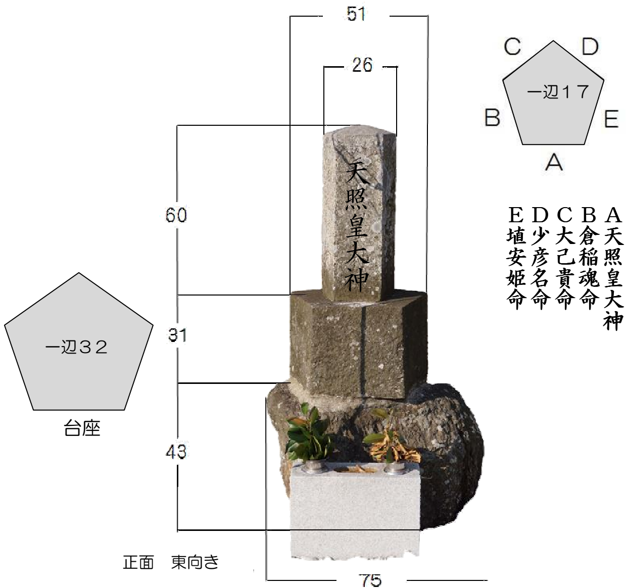
福吉地神様寸法図（単位：cm）
