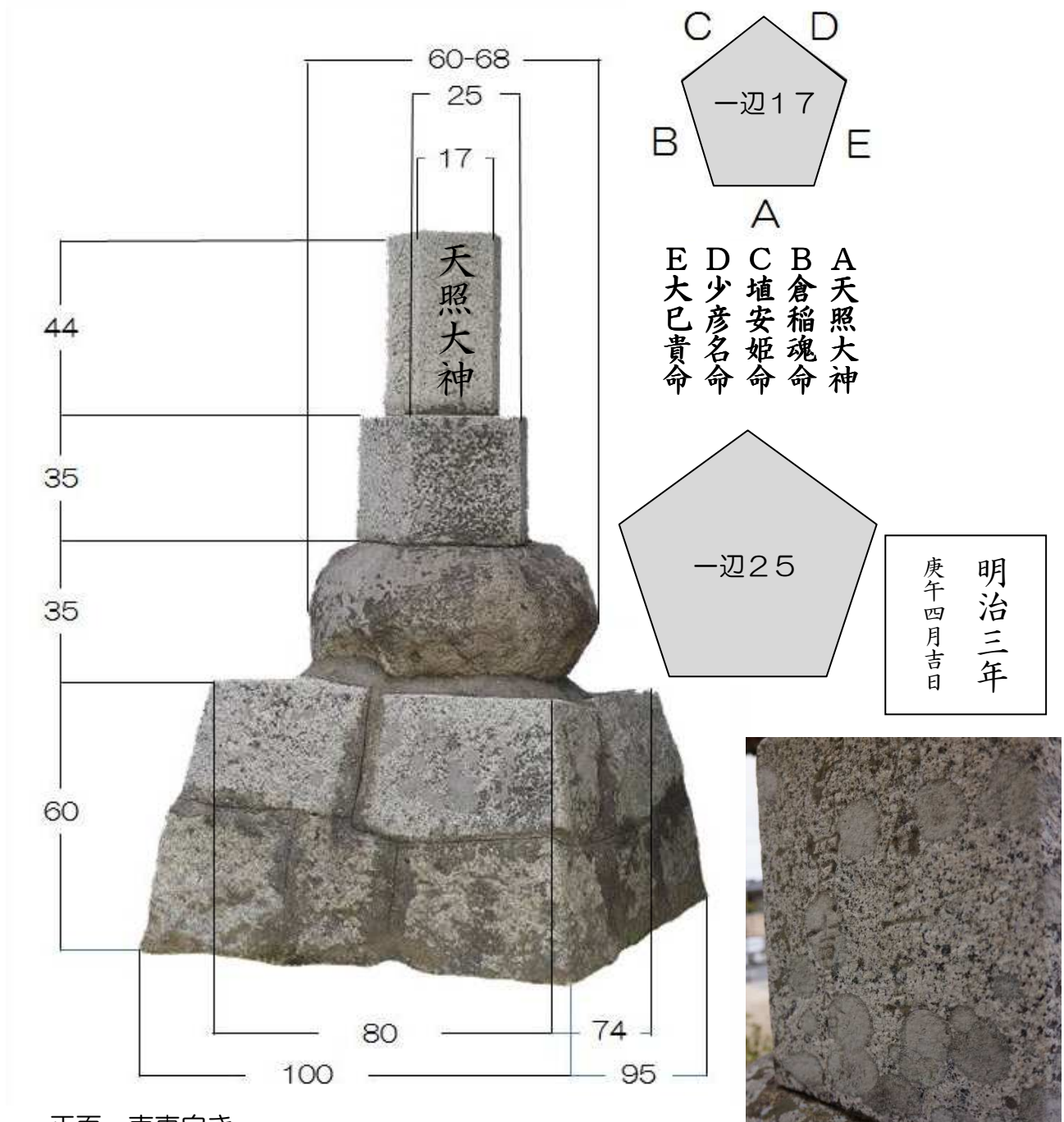
出村地神様寸法図（単位：cm）
