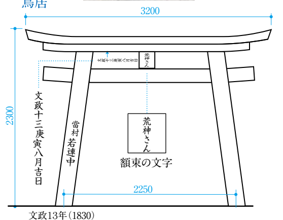
鳥居断面
