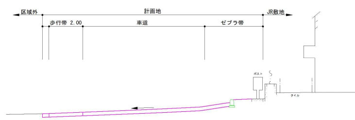
②-②断面図（駅前交差点）
