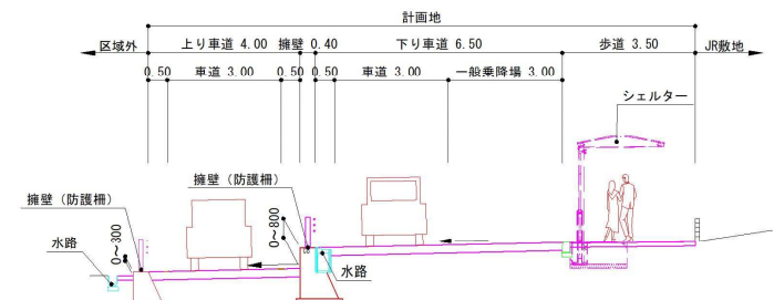
①-①断面図（一般車側）
