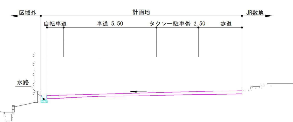
③-③断面図（タクシー乗降側）
