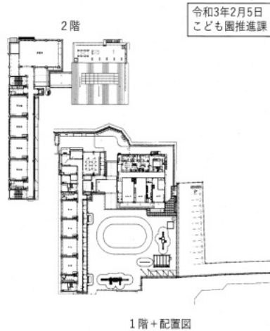
陵南幼稚園・子ども園完成見取図
