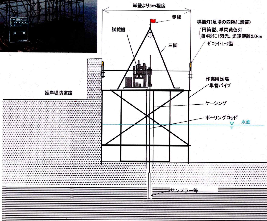
図 2 ボーリング作業足場の仮設イメージ図
